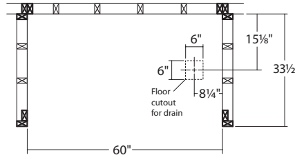
6030 Elite™ RH Drain (LEBxx6030R) 6030 Elite™ LH Drain (LEBxx6030L)
